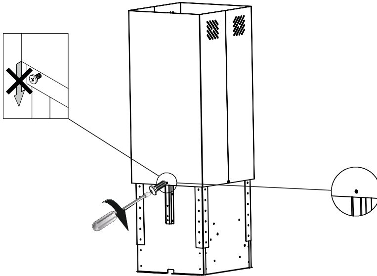
Gösterildiği şekilde İç Bacanın Yüksekliği Ayarlanarak Sabitlenir.
